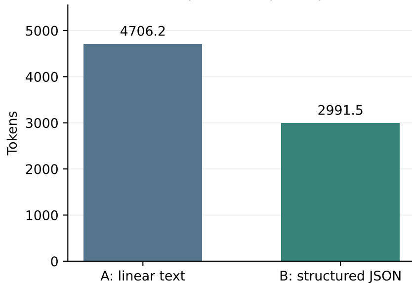
Mean input tokens per request
