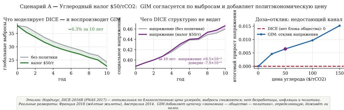
Рис. 6: Сценарий углеродного налога. Слева: GIM воспроизводит снижение выбросов, которое моделирует DICE. В центре: GIM добавляет рост социального напряжения, недоступный DICE. Справа: зависимость отклика напряжения от ставки налога имеет ненулевой наклон у GIM против нулевого отклика у DICE.
