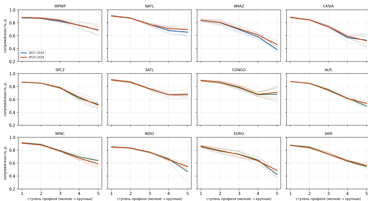
Рис. 1. Профили сопряжённости уровней P для двенадцати основных областей (коды – табл. 1): тонкие линии – отдельные сезонные окна, жирные – средние по периодам 2017–2019, 2021–2022 и 2023–2024 гг. Ступени 1–5 отвечают парам соседних уровней от (мельче 50; 50–100 км) до (400–800; 800–1600 км).
