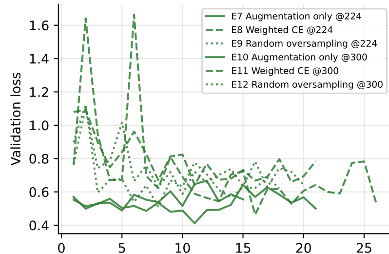
EfficientNet-B3
