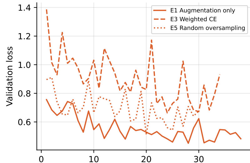
MobileNetV2
