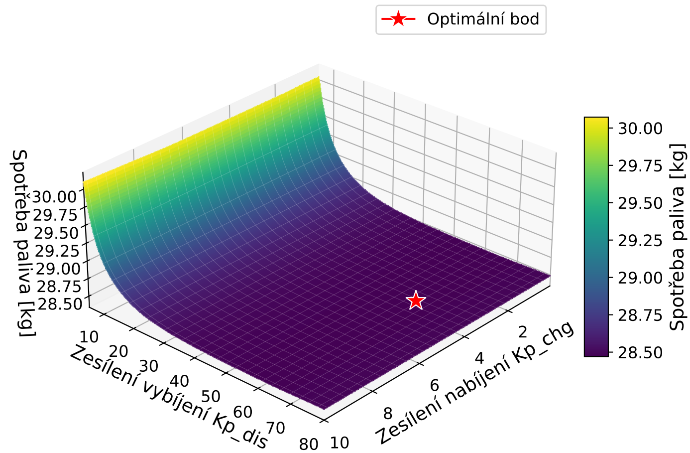
A-ECMS 3D optimalizační plocha
