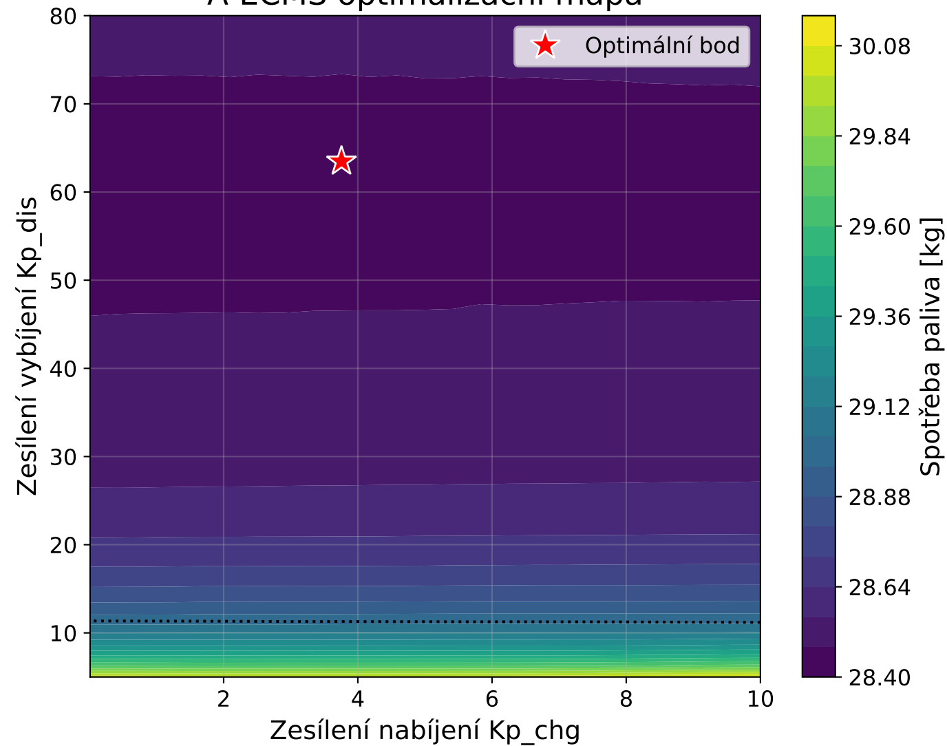
A-ECMS optimalizační mapa
