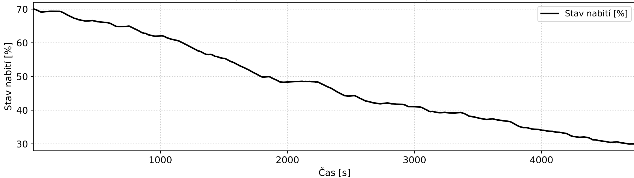
Strategie: ECMS | Kapacita baterie: 120.0 kWh | Palivo: 27.984 kg
