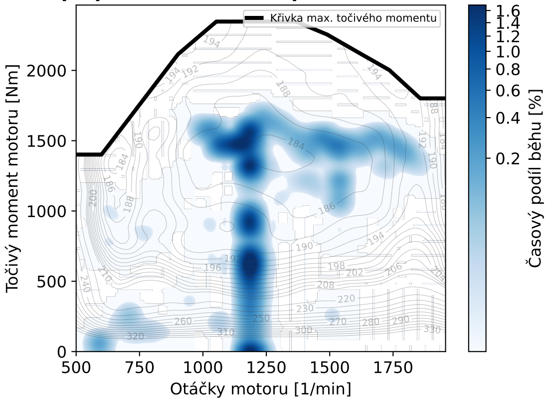
Mapa provozních bodů spalovacího motoru
