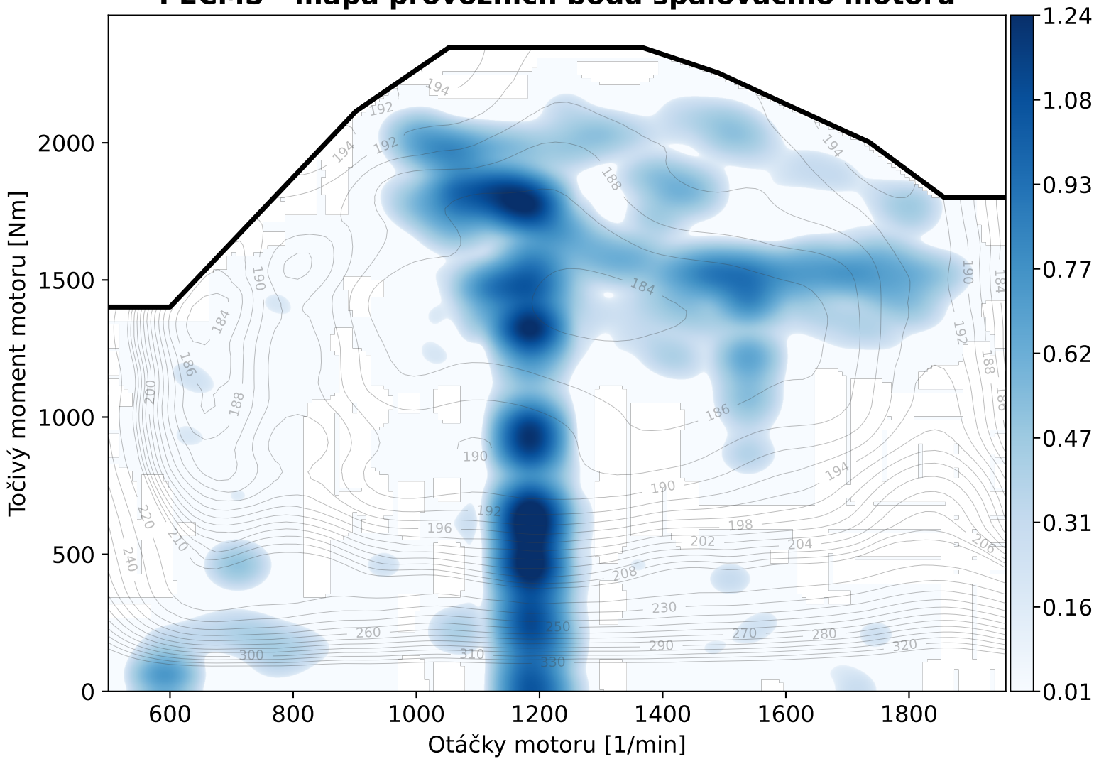
PECMS - mapa provozních bodů spalovacího motoru
