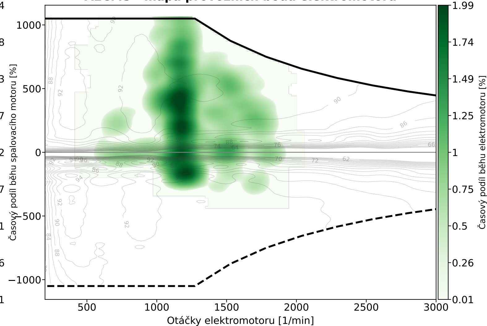
AECMS - mapa provozních bodů elektromotoru
