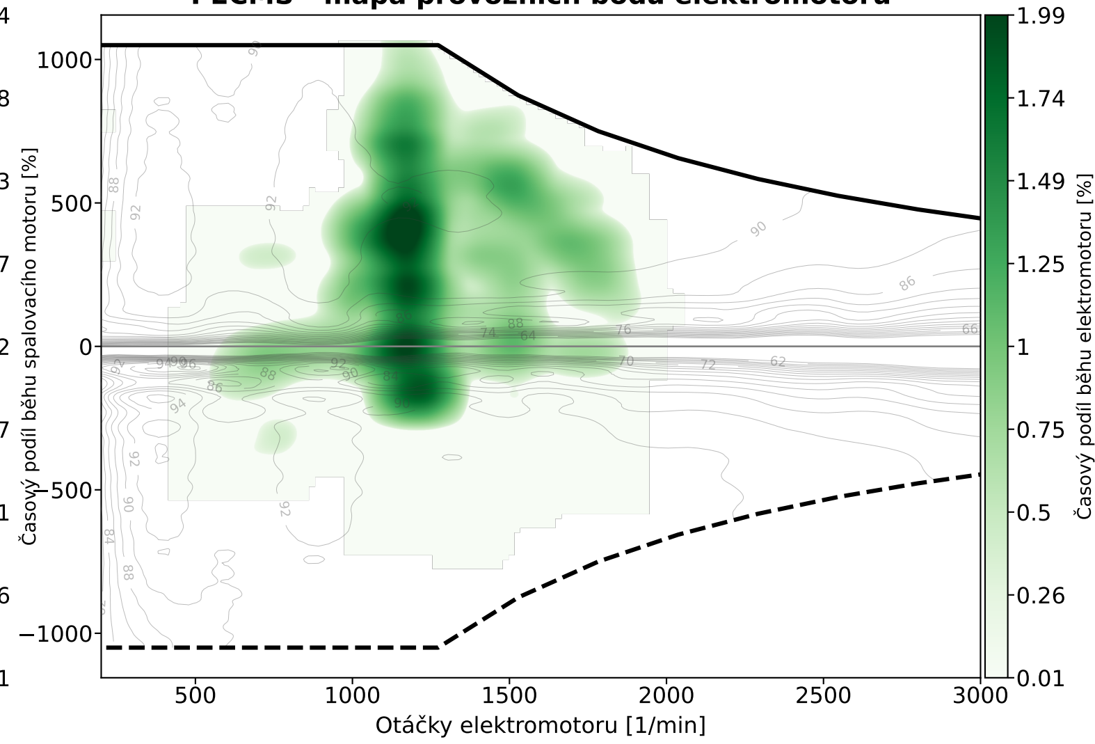
PECMS - mapa provozních bodů elektromotoru
