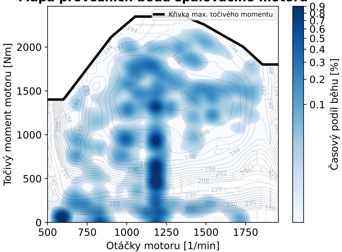
Mapa provozních bodů spalovacího motoru
