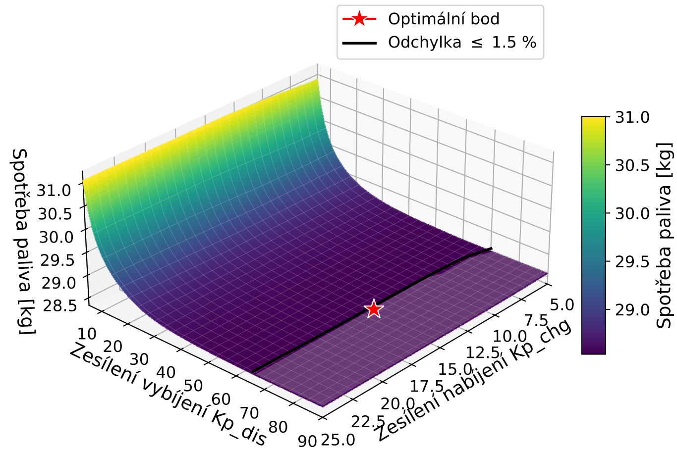
A-ECMS 3D optimalizační plocha
