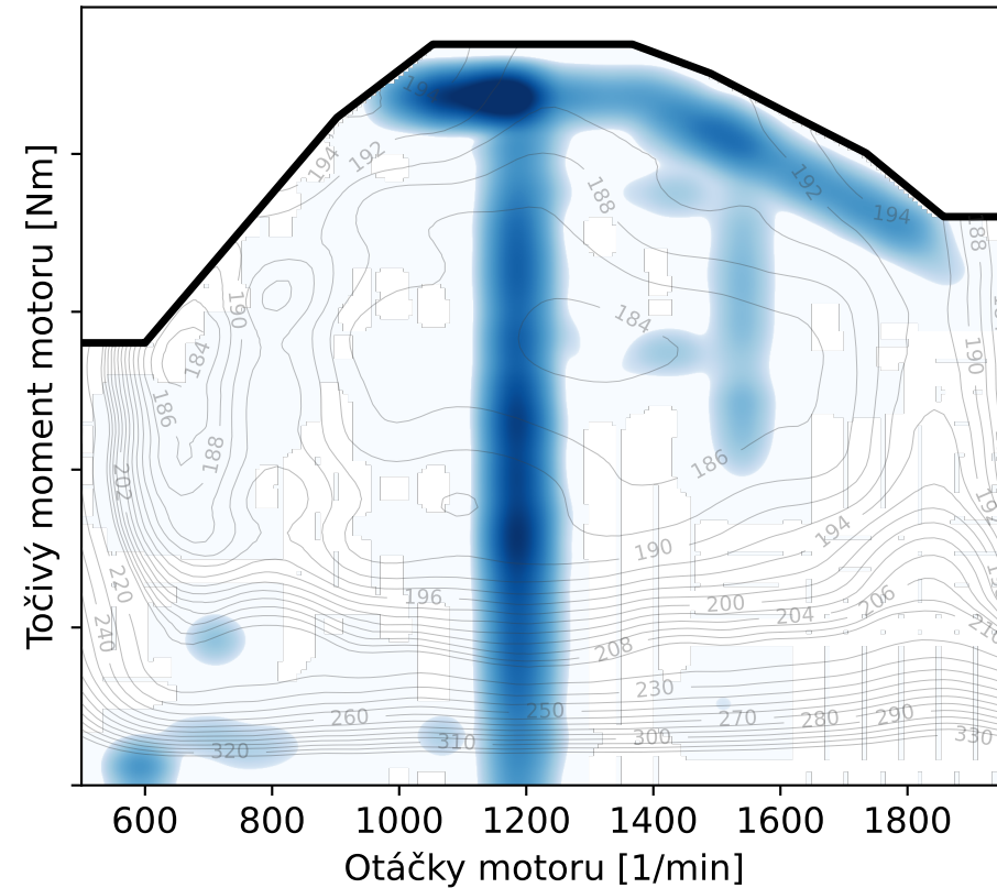
Točivý moment motoru [Nm]
