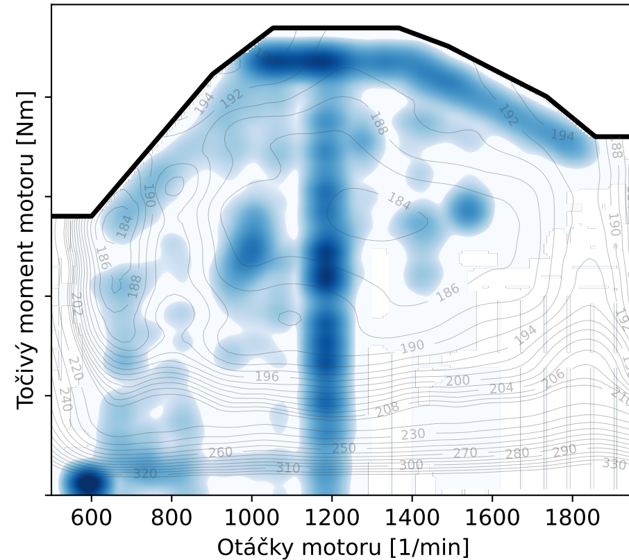
(b) Pouze ICE na mapě BSFC
