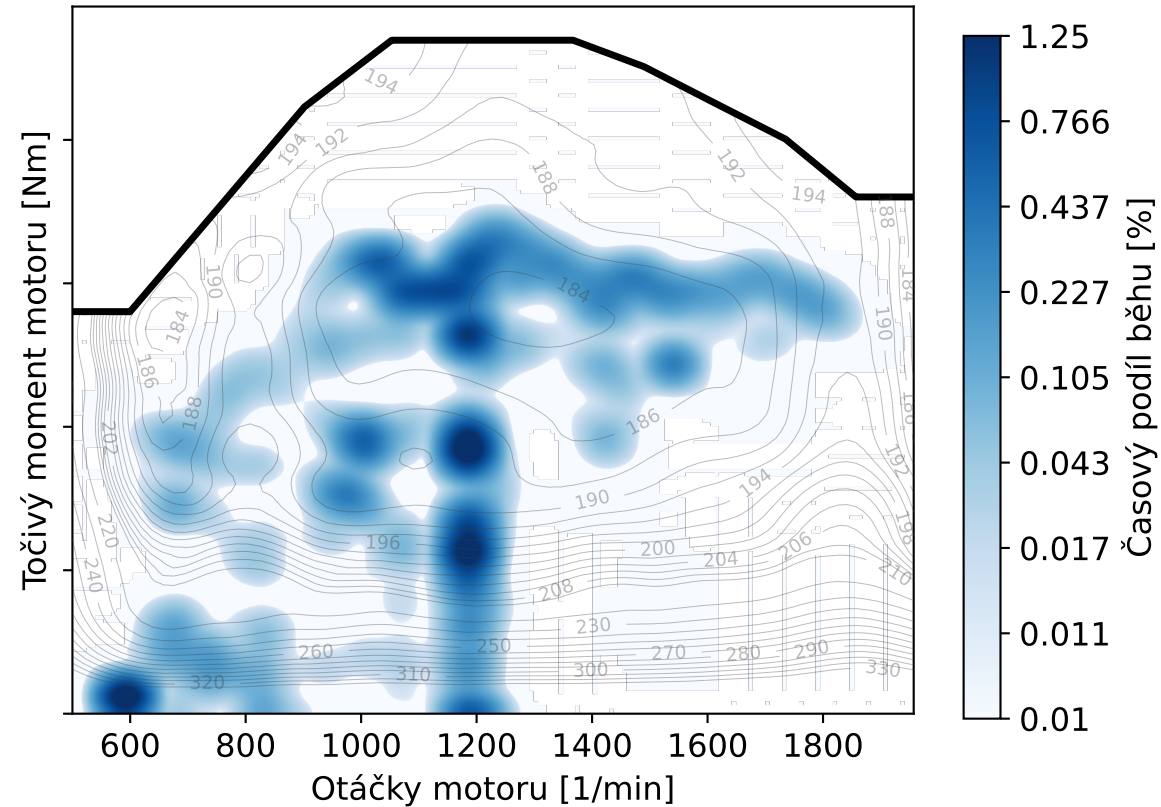
(c) ECMS na mapě BSFC
