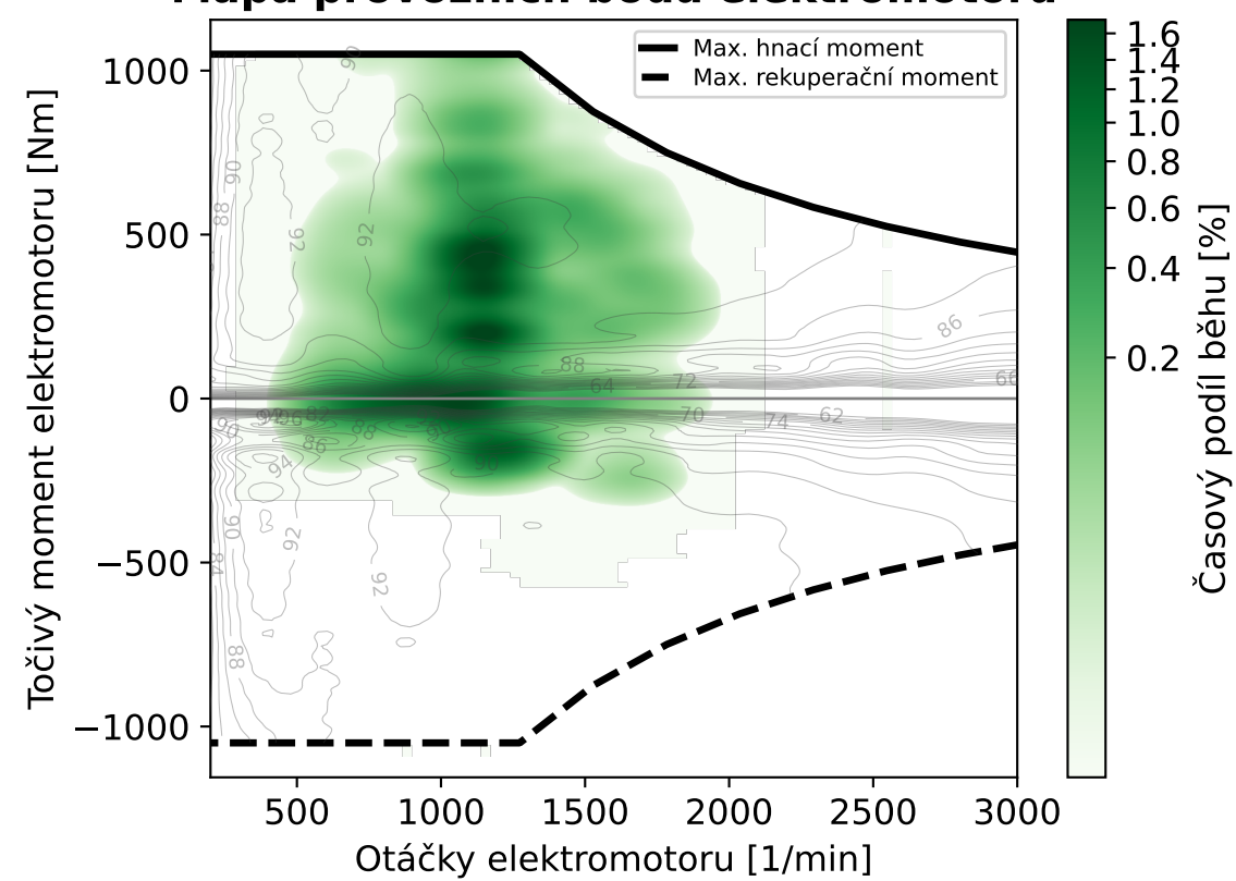
Mapa provozních bodů elektromotoru
