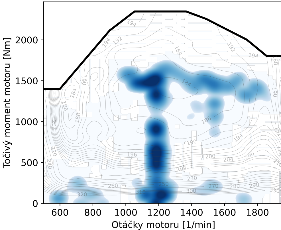
(a) DP na mapě BSFC
