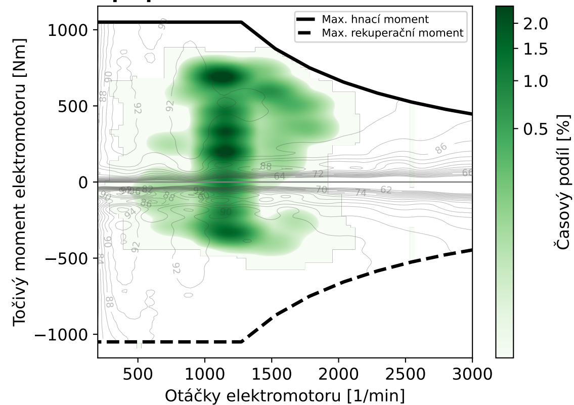
Mapa provozních bodů elektromotoru
