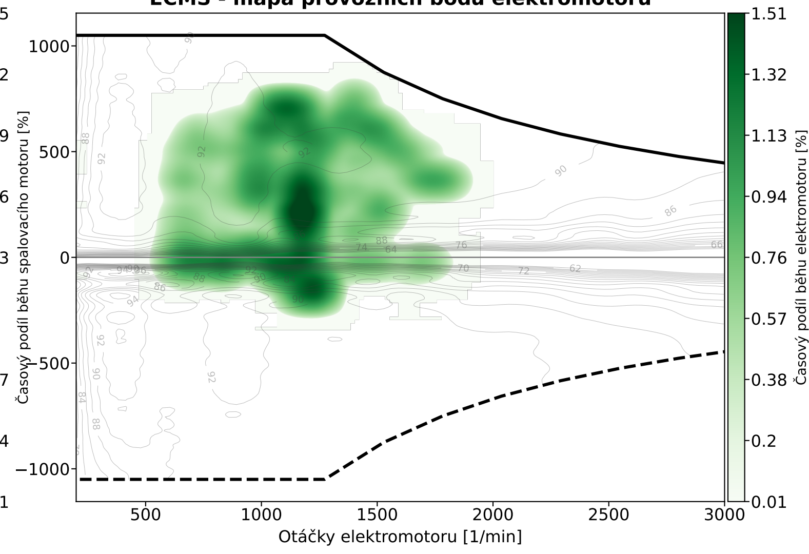
ECMS - mapa provozních bodů elektromotoru
