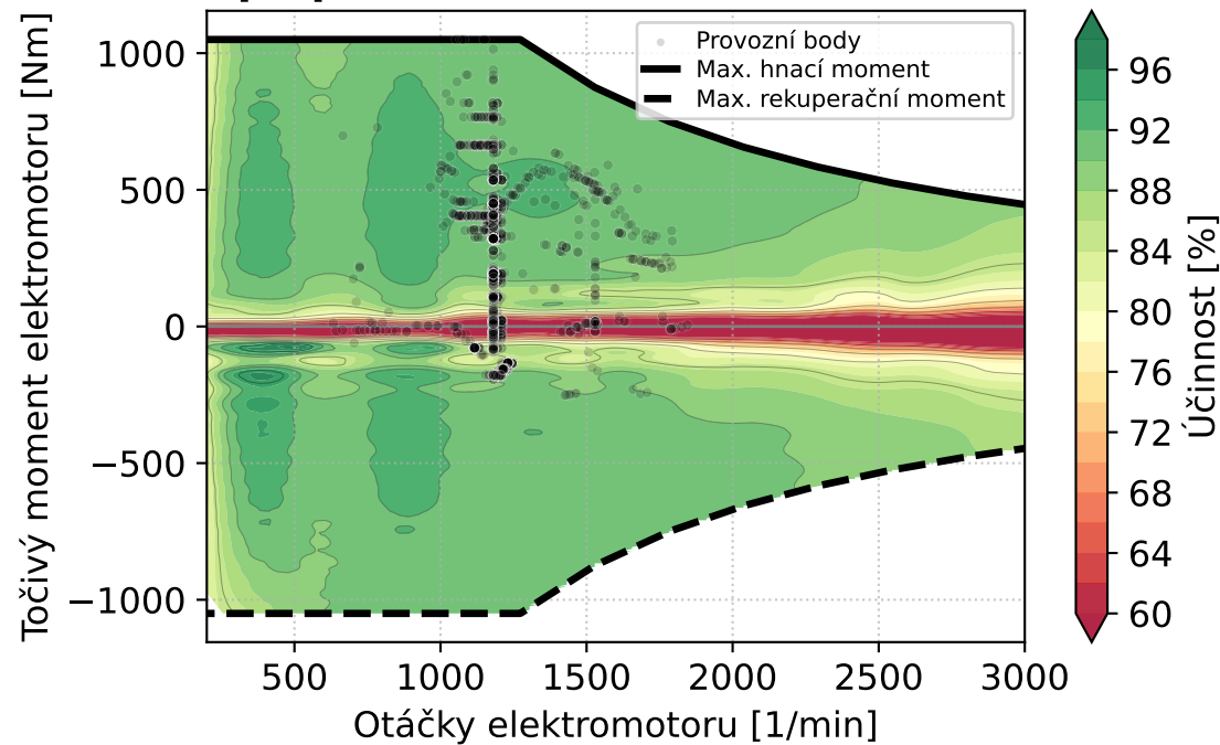
Mapa provozních bodů elektromotoru
