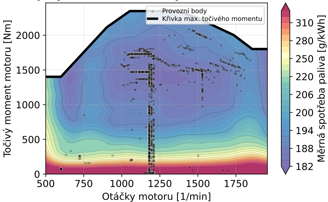
Mapa provozních bodů spalovacího motoru
