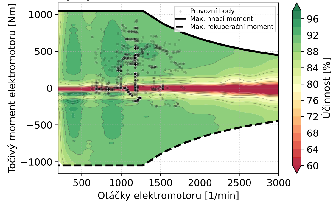
Mapa provozních bodů elektromotoru
