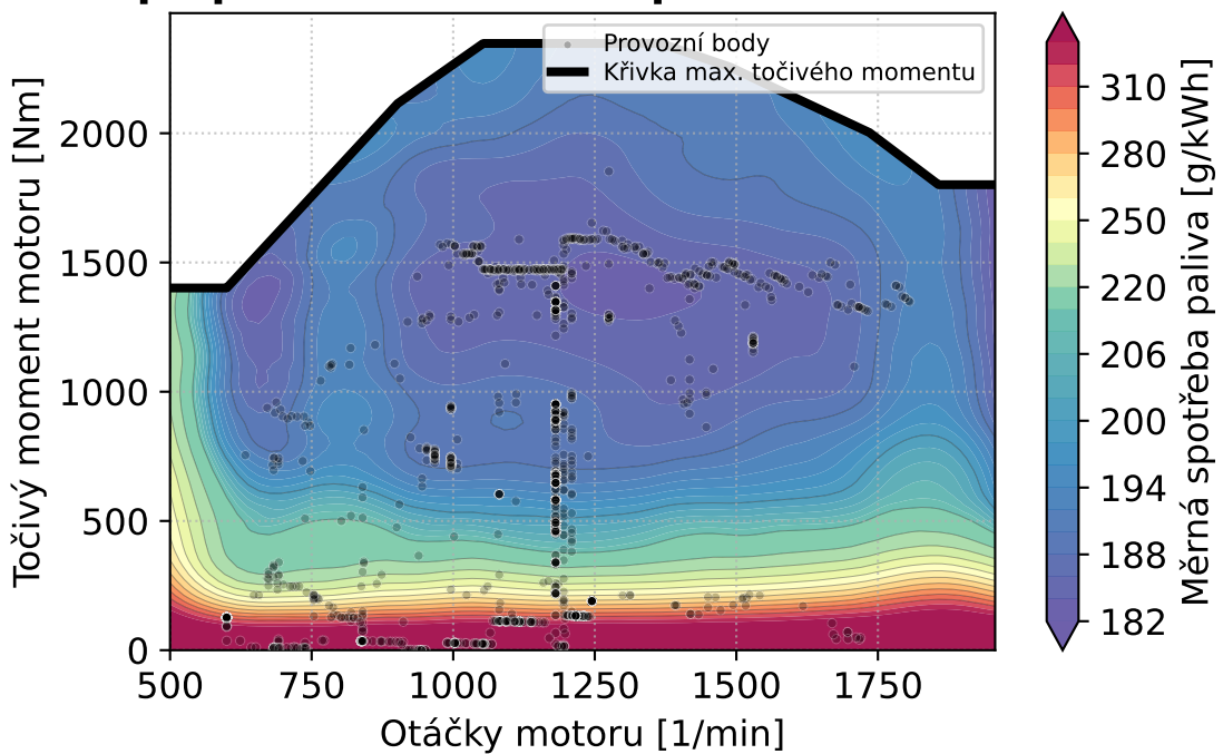
Mapa provozních bodů spalovacího motoru
