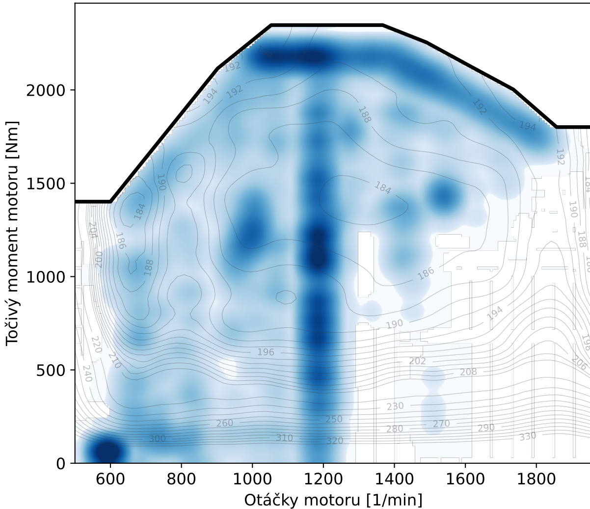
(a) Pouze ICE na mapě BSFC
