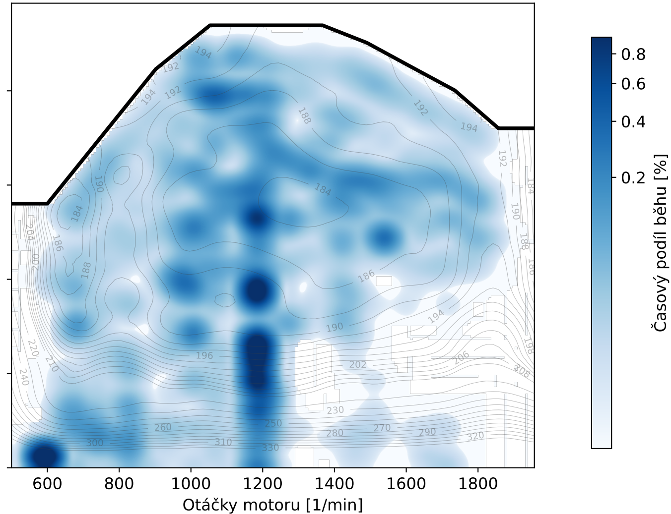
(b) PECMS na mapě BSFC
