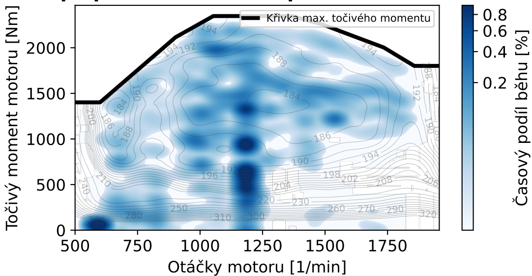
Mapa provozních bodů spalovacího motoru
