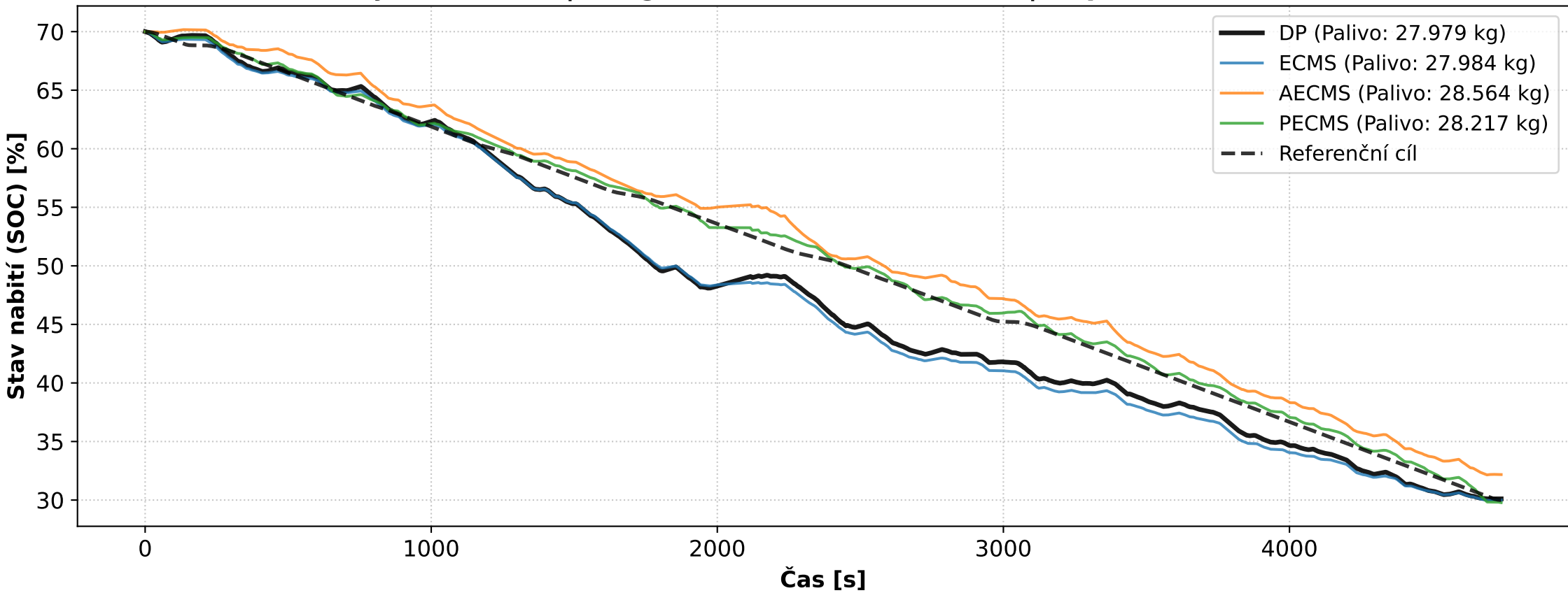
Porovnání trajektorií SOC | LongHaulEMSReferenceLoad | Kapacita baterie: 120.0 kWh
