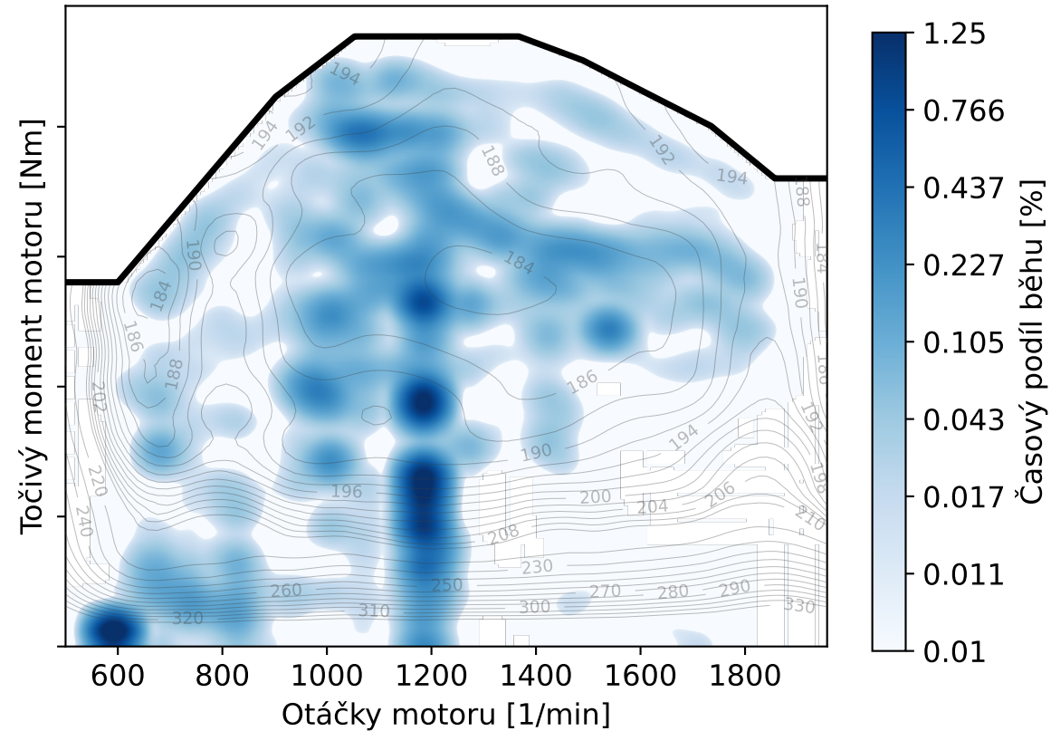
(c) PECMS na mapě BSFC
