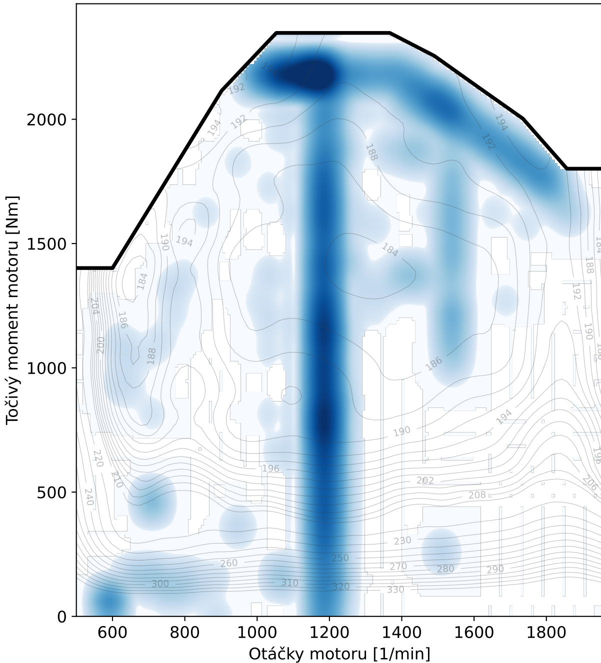
(a) Pouze ICE na mapě BSFC
