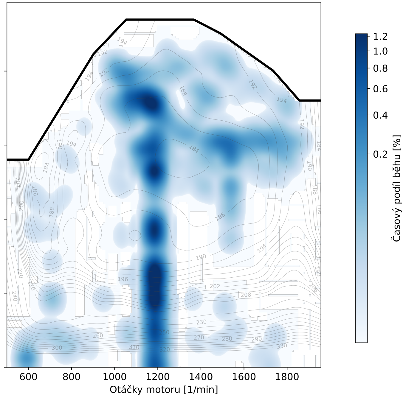
(b) PECMS na mapě BSFC
