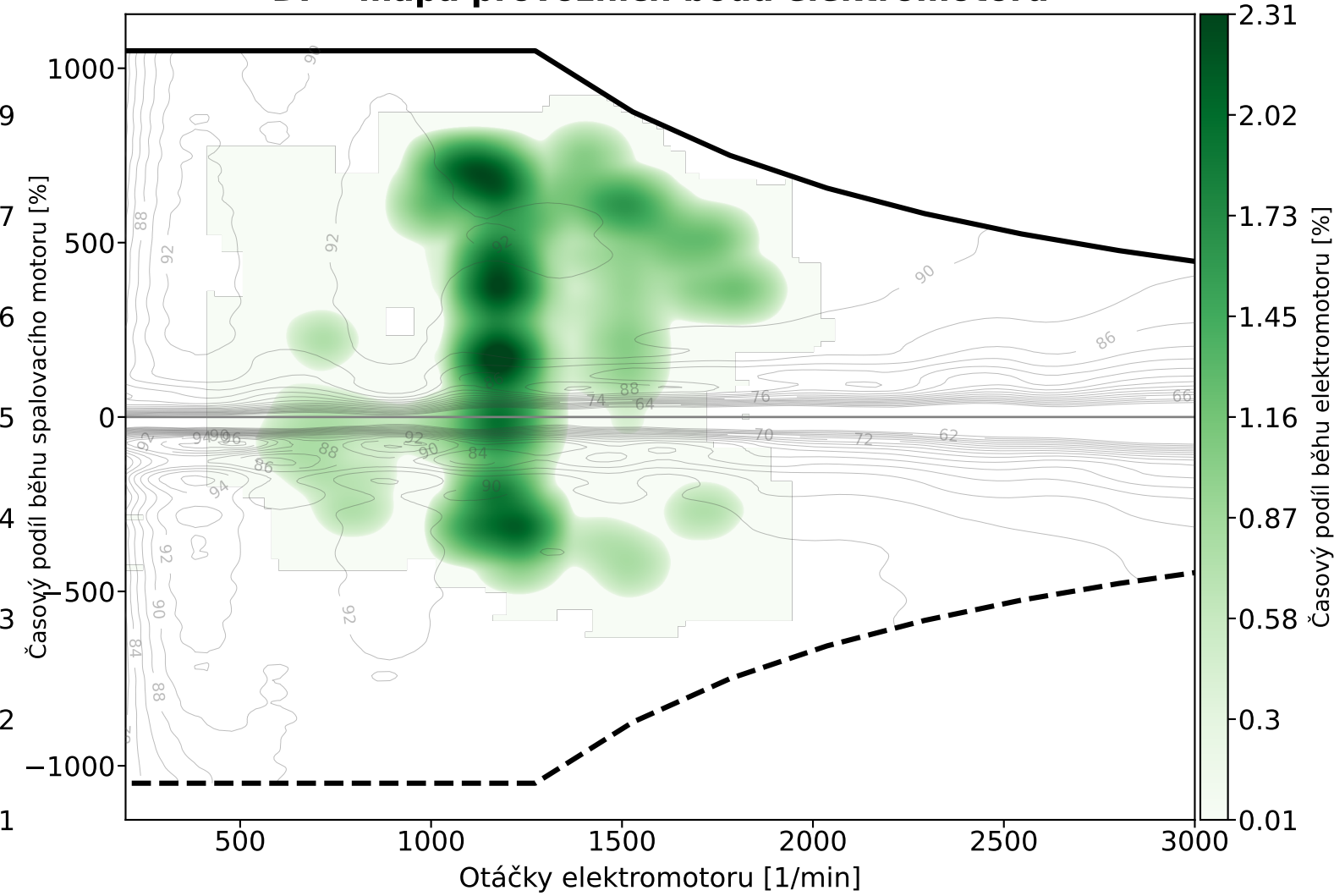
ECMS - mapa provozních bodů elektromotoru
