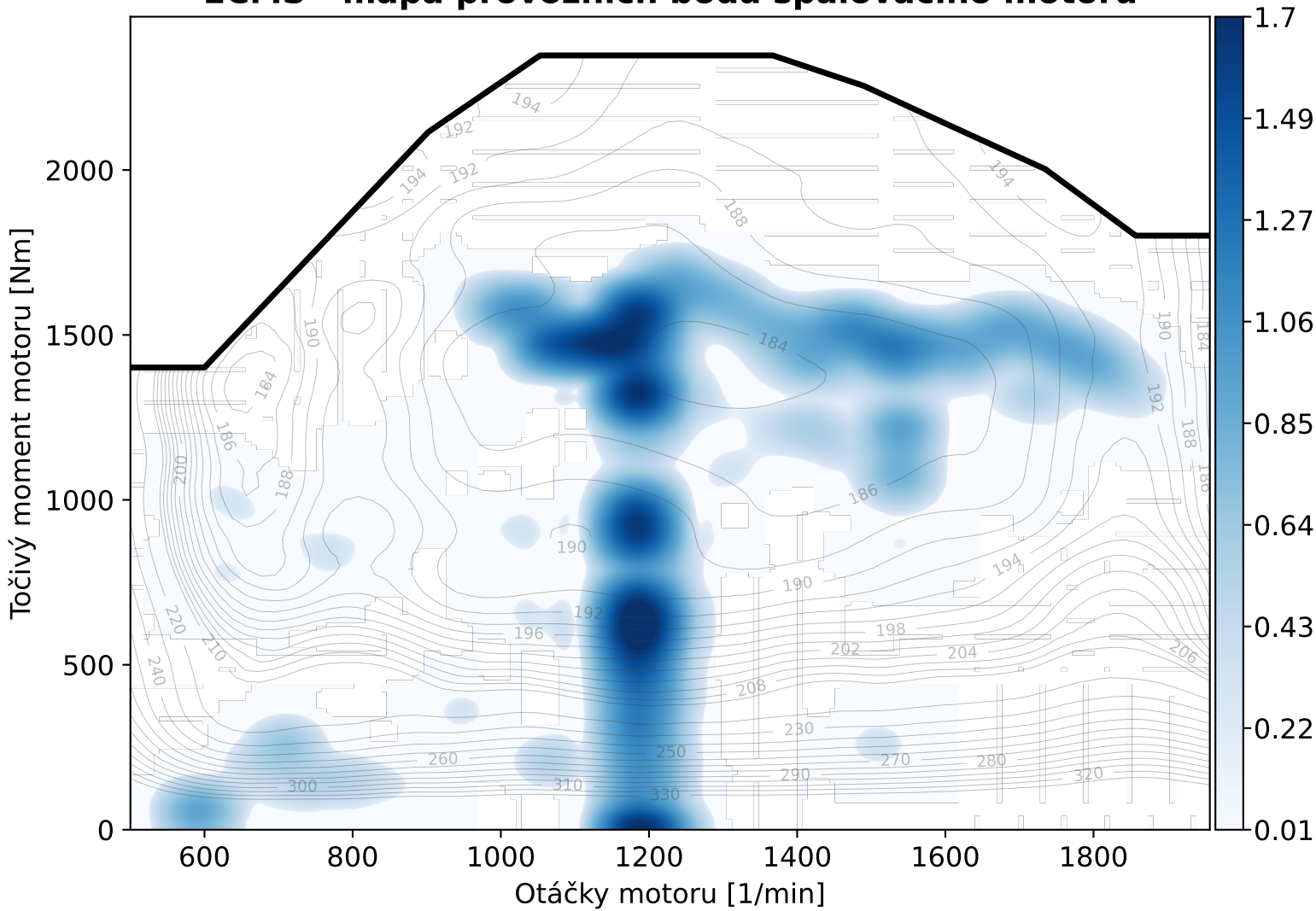
ECMS - mapa provozních bodů spalovacího motoru
