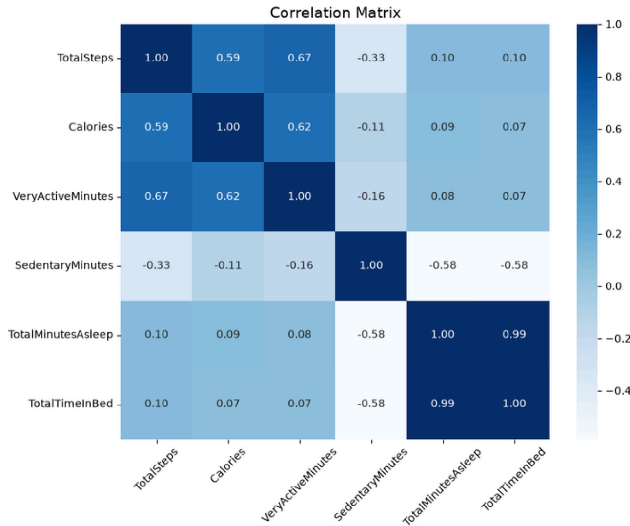
Gráfica 5 Matriz de correlación.
