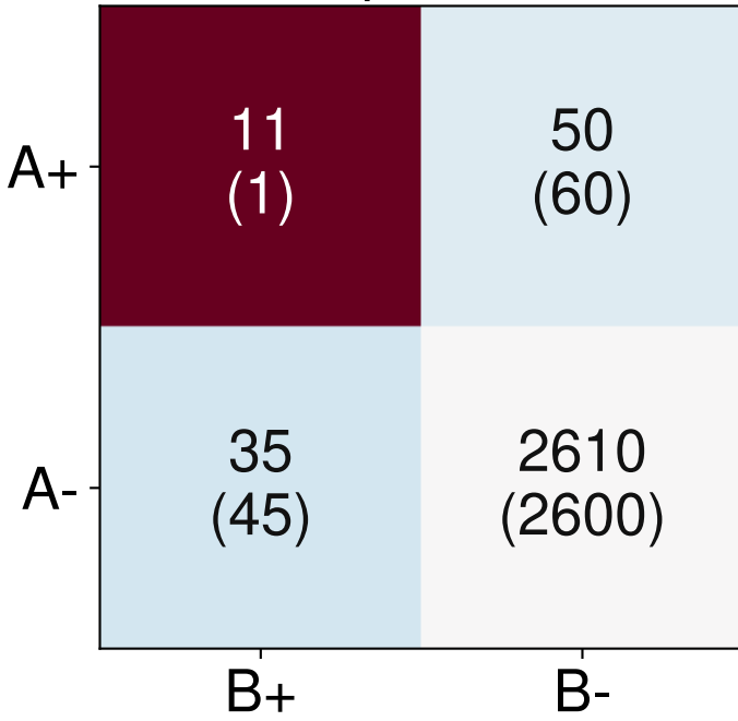
PCID2 axa d=38bp OR=16.7
