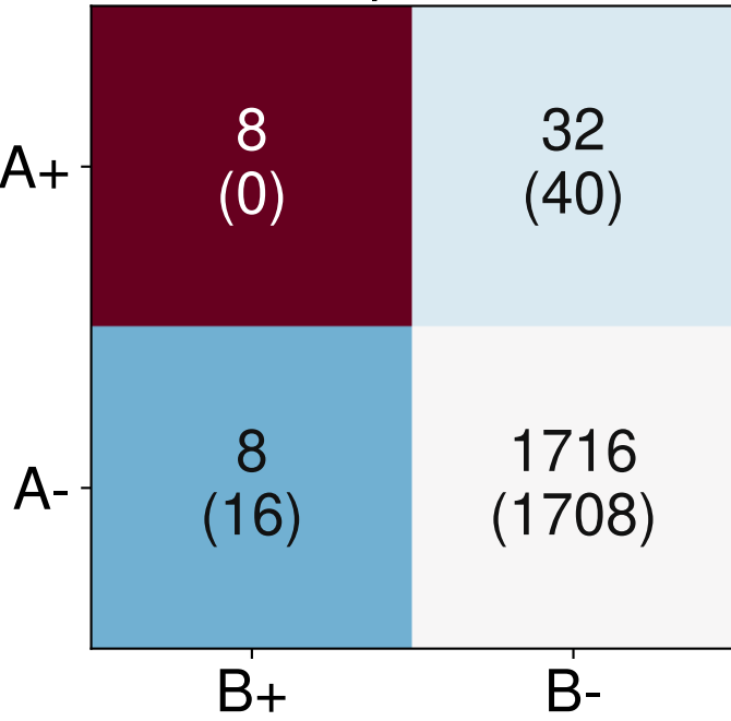
PCID2 axa d=355bp OR=52.8
