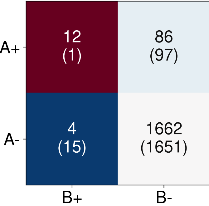
PCID2 axa d=63bp OR=11.9
