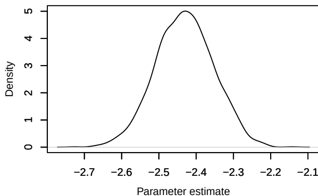
Density – loglik[223]
