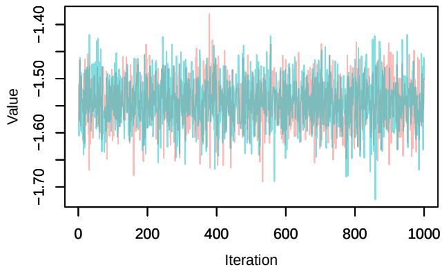
Trace – loglik[258]
