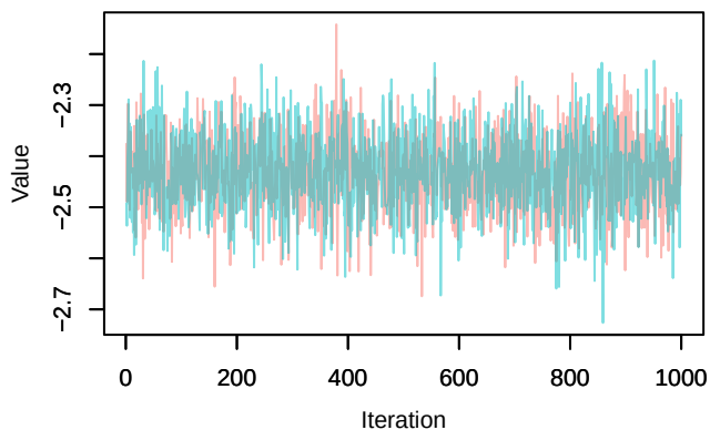
Trace – loglik[223]
