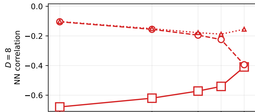
Dimer-plaquette pin
