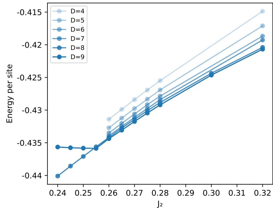
C6Y \pi
