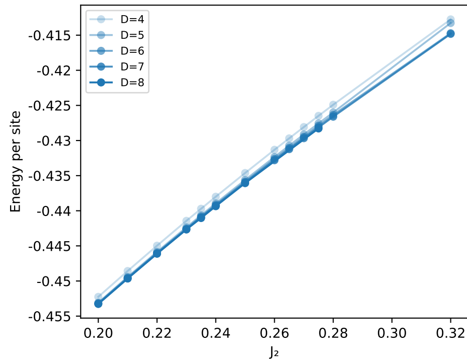
Néel
