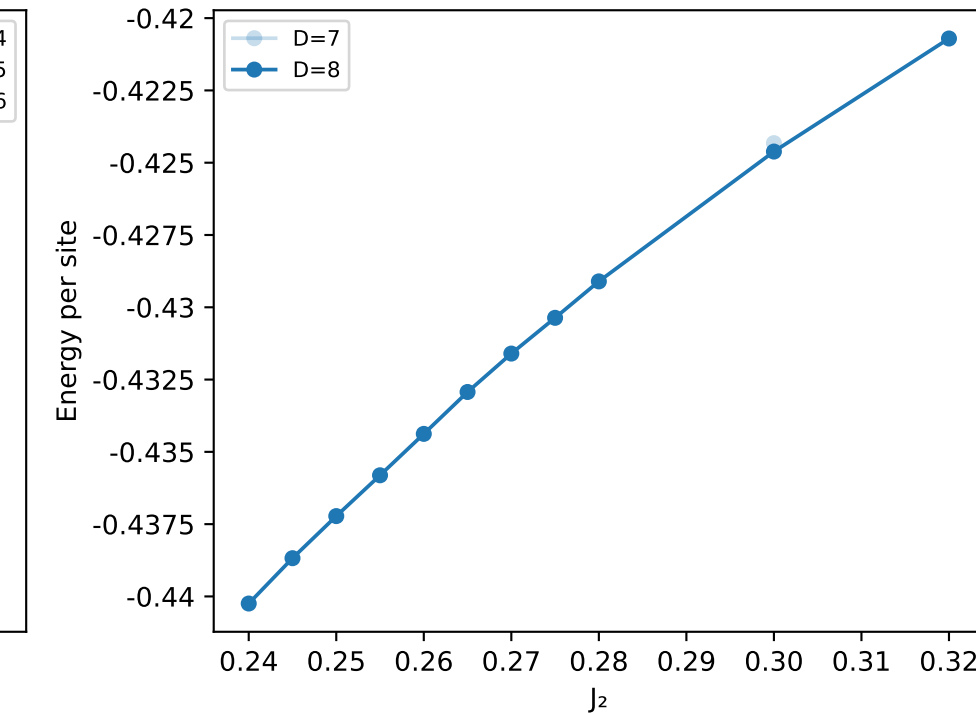
2 C3
