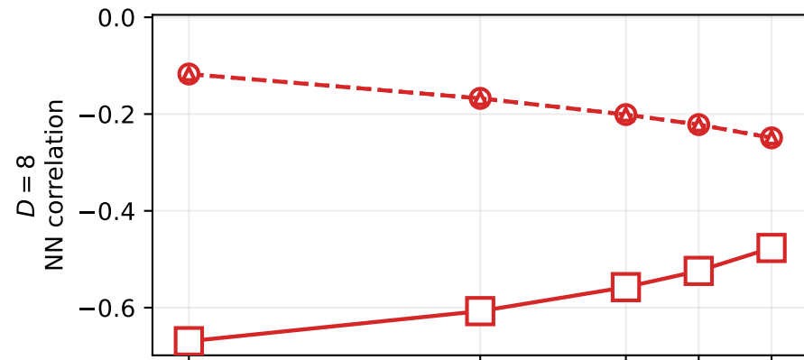
Dimer-plaquette pin
