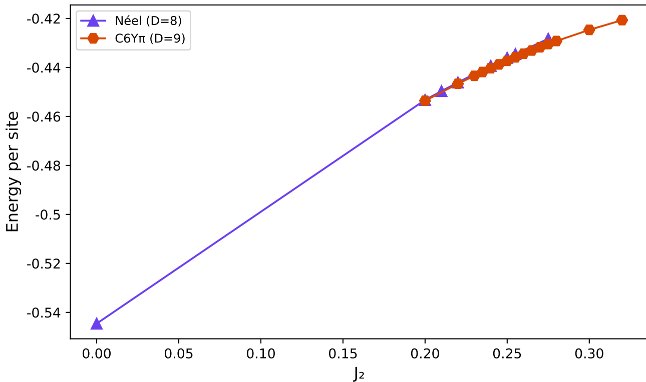
Energy: Néel (D=8) vs C6Y \pi (D=9)
