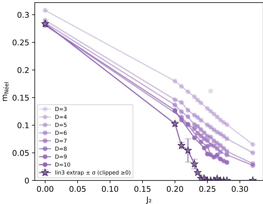
Néel
