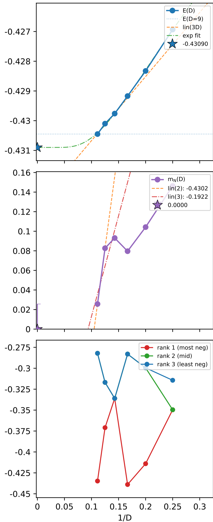
C6Y \pi
