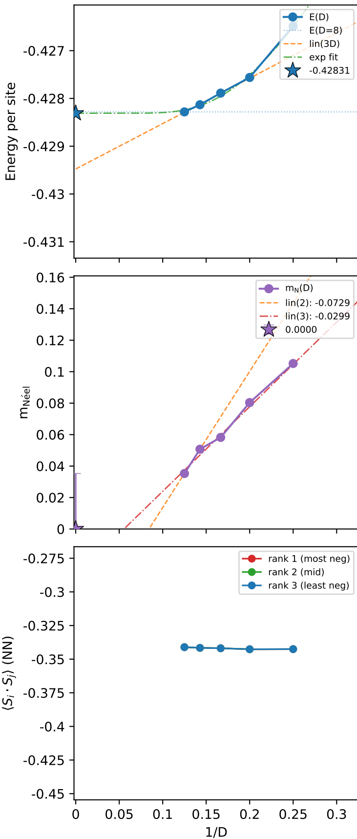
Néel
