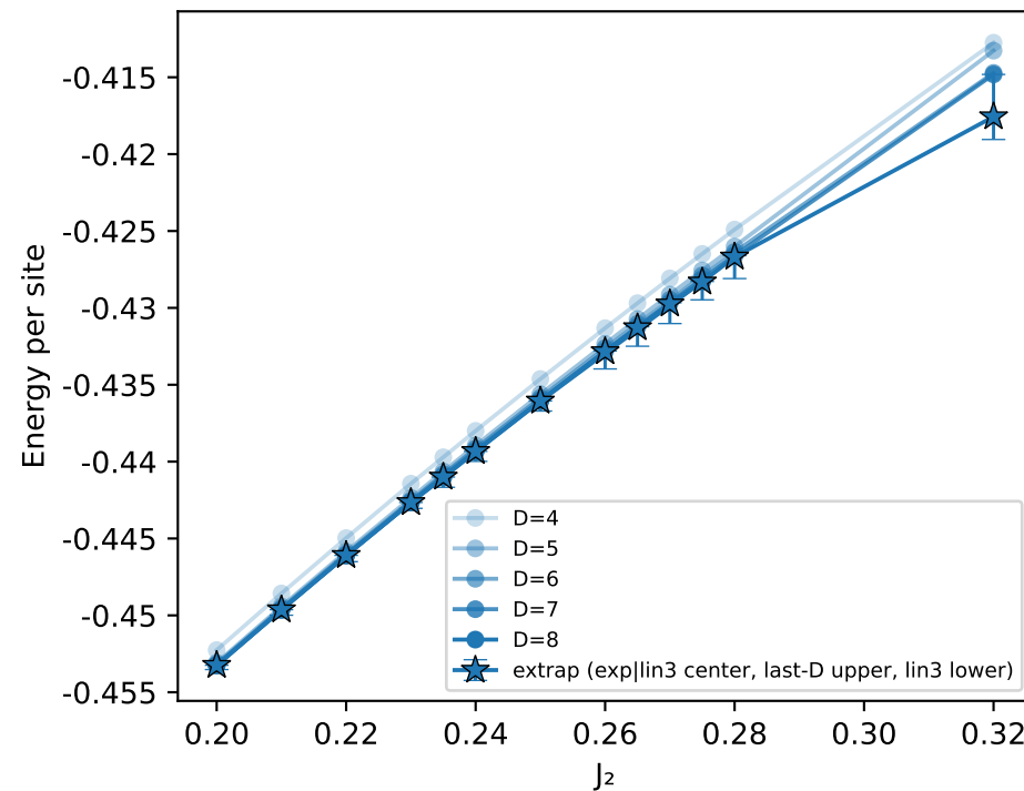
Néel
