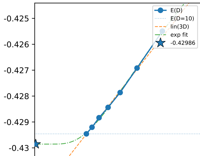
C6Y \pi
