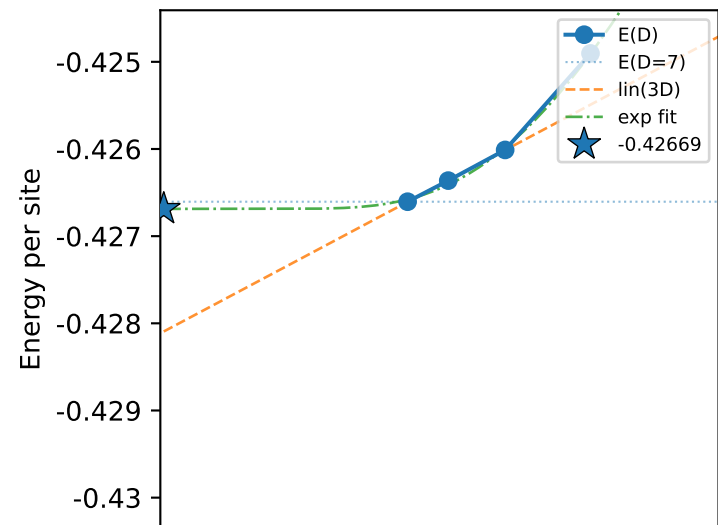
Néel
