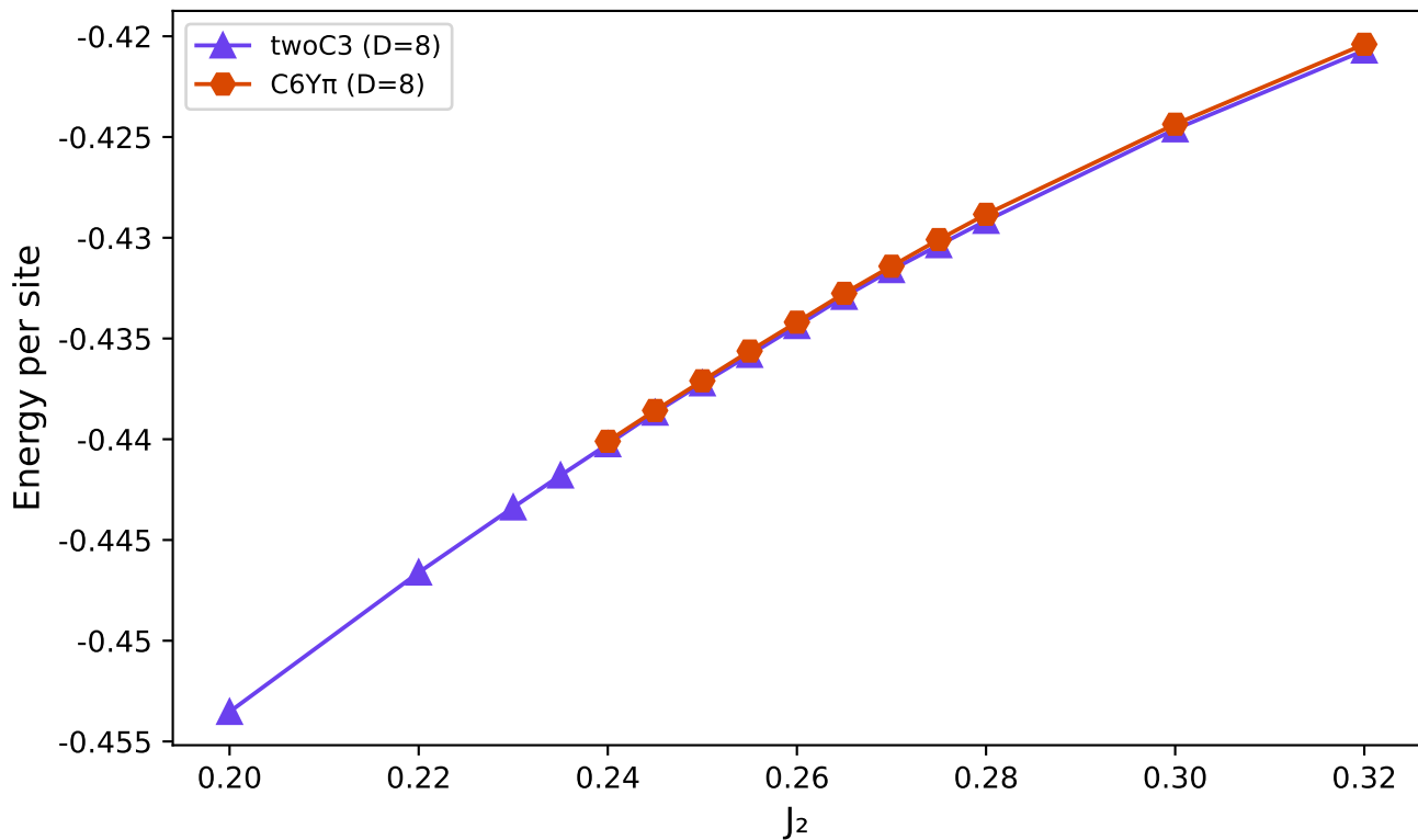
Energy: twoC3 (D=8) vs C6Y \pi (D=8)
