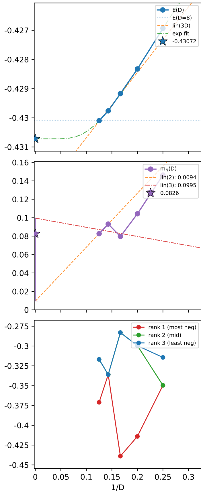
C6Y \pi
