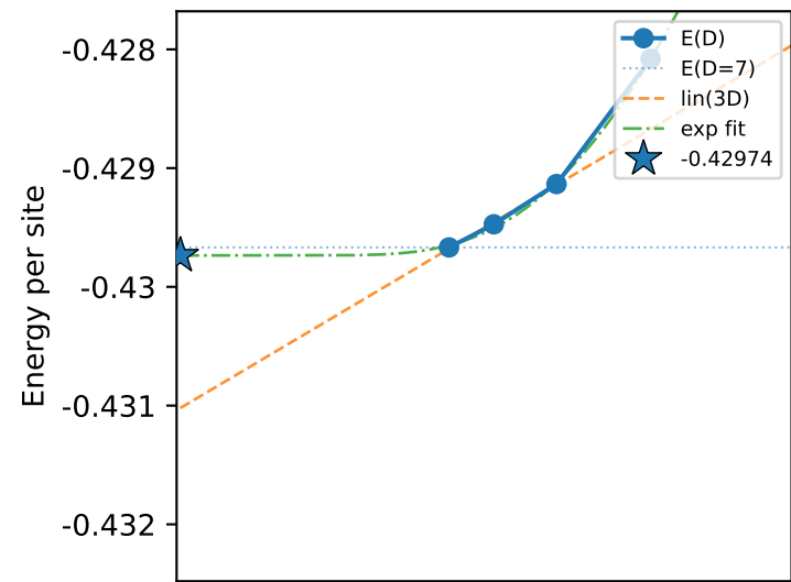
Néel
