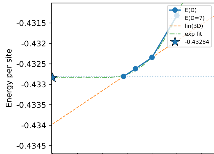
Néel
