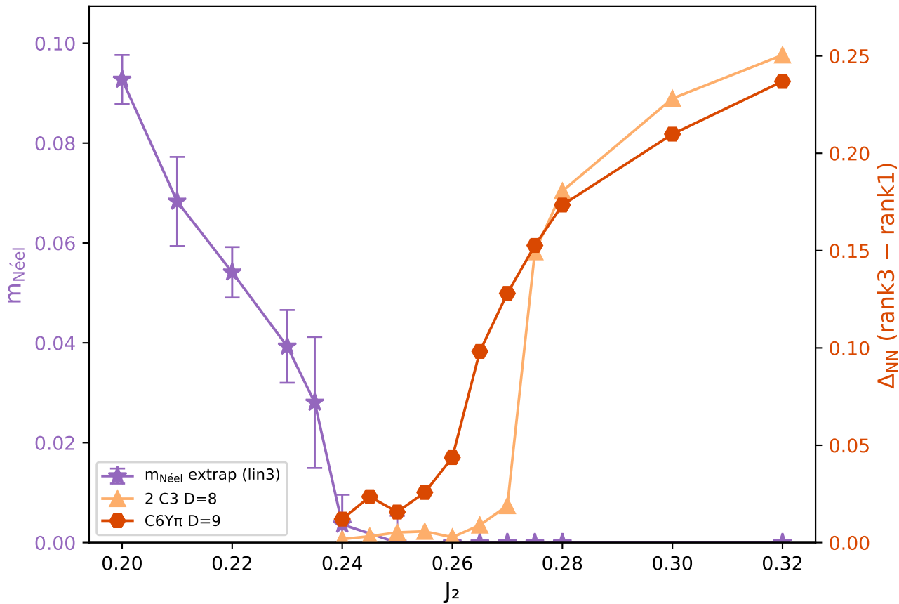
Néel m_{\text{Néel}} extrap & NN splitting ( 0.20 \leq J_2 \leq 0.32 )
