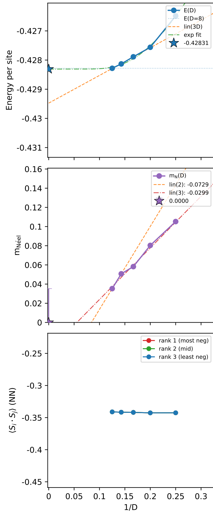
Néel
