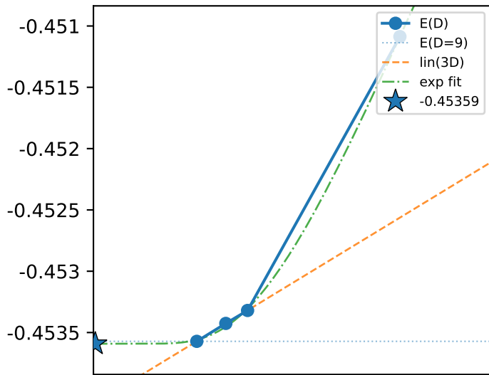
C6Y \pi
