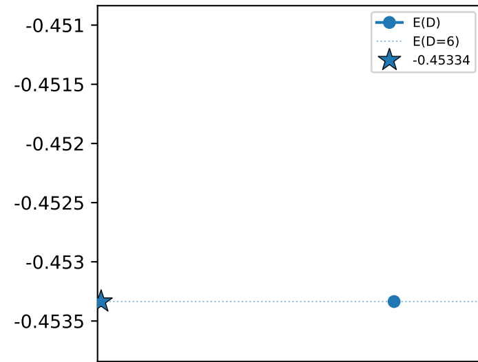
2 C3
