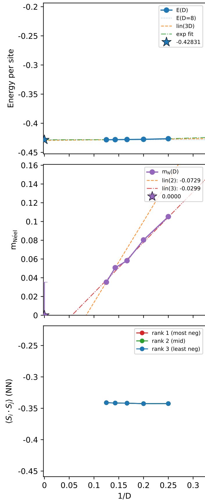
Néel
