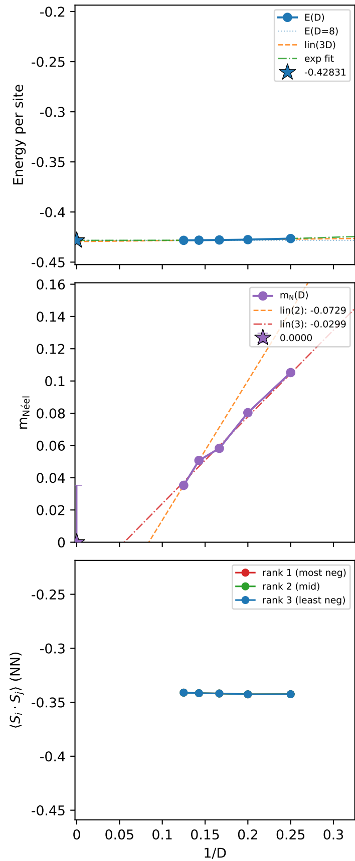
Néel
