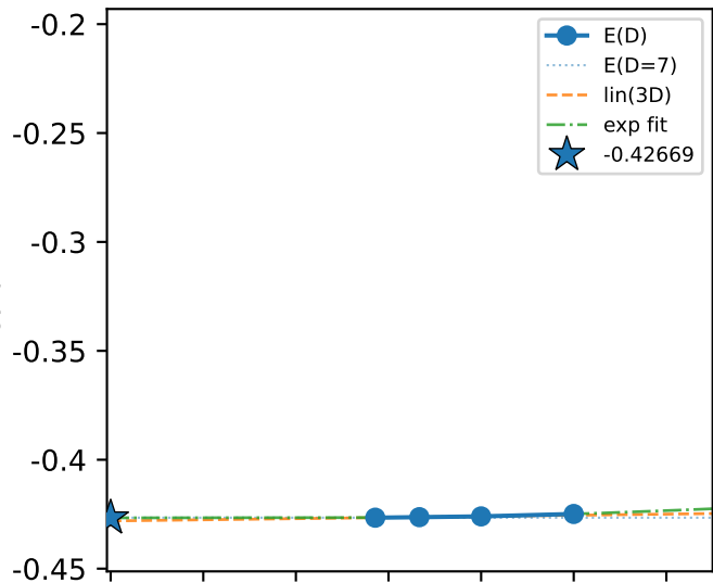
Néel
