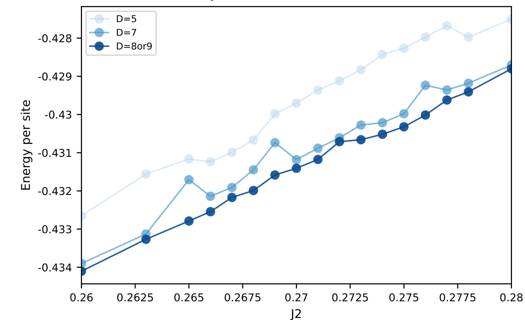
Zoom J_2 \in [0.26, 0.28] ( D=5 , D=7 , D=8 or 9 )
