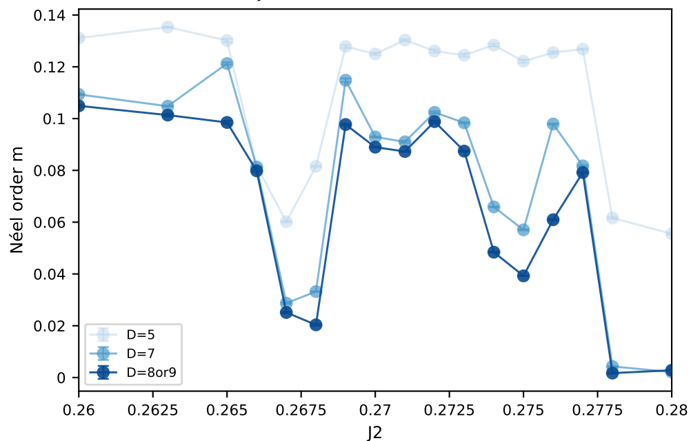
Zoom J_2 \in [0.26, 0.28] ( D=5 , D=7 , D=8 or 9 )
