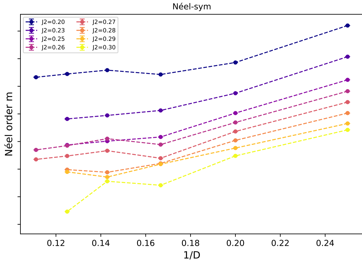
Néel order parameter m vs 1/D
