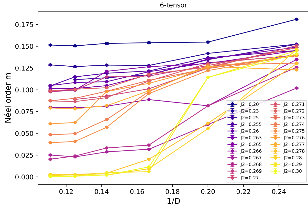
Néel order parameter m vs 1/D
