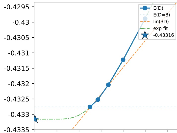
C6Y \pi
