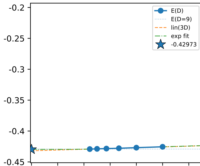
C6Y \pi
