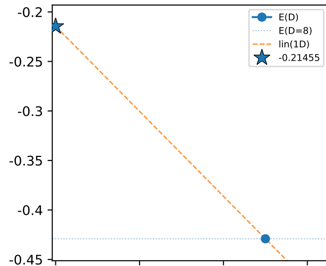
2 C3
